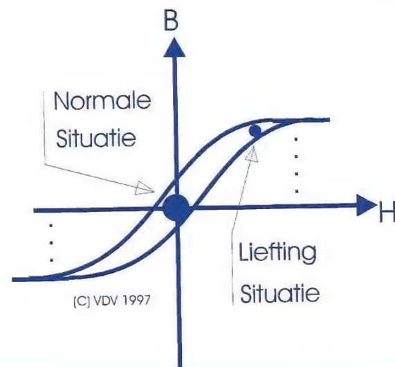
Figuur 5 Rustpositie op de magnetisatiecurve van de uitgangstransformator; De "Liefting"-situatie zit vlak bij de verzadigingsgrens.
